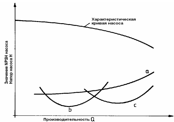
Рис. 33. Характеристика NPSH_{eff} со стимулятором (предвключённым ротором) и без него
