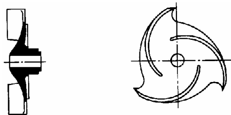
Открытое трёхлопастное колесо
