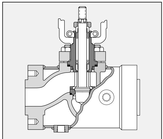
Рисунок 6: Клапан с паровой рубашкой
