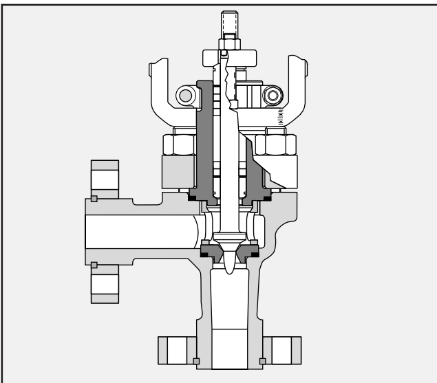
Рисунок 5: Угловой клапан
