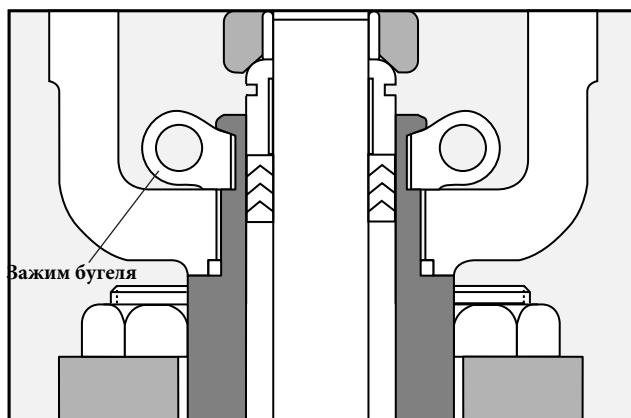
Рисунок 10: Зажим бугеля
