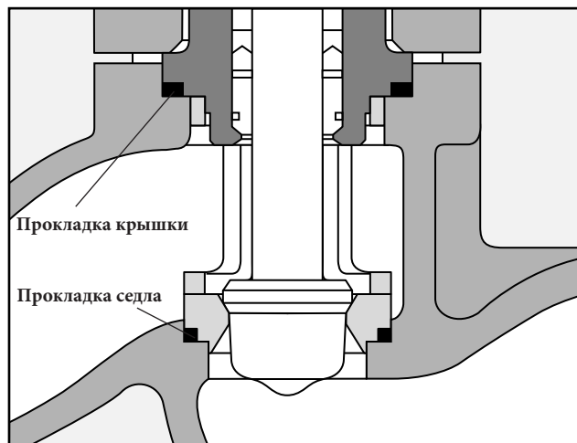
Рисунок 9: Прокладки корпуса
