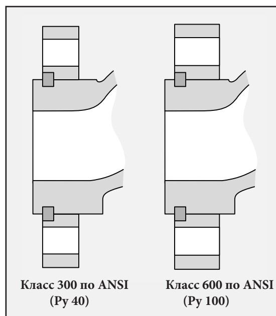
Рисунок 8: Присоединительные фланцы
