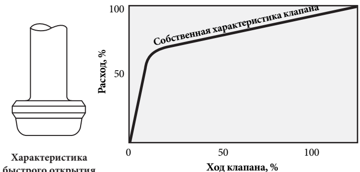
Рисунок 13: Расходные характеристики
