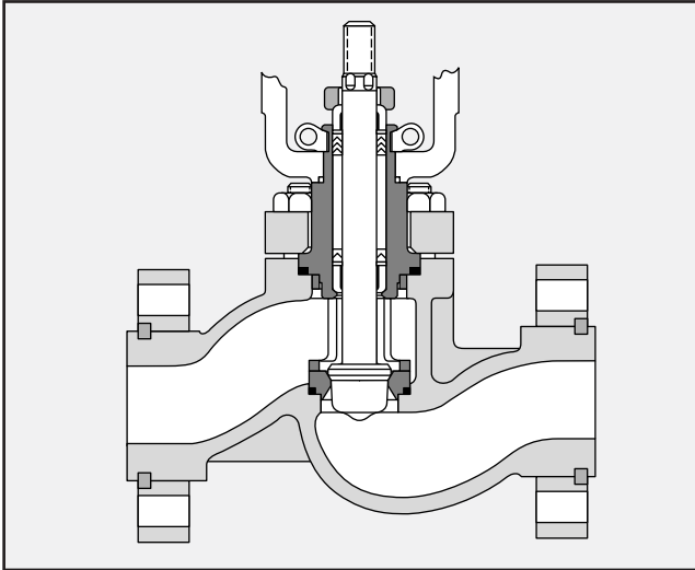
Рисунок 3: Прямой клапан
