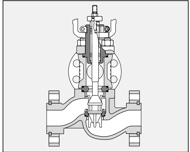
Рисунок 4: Трехходовой клапан
