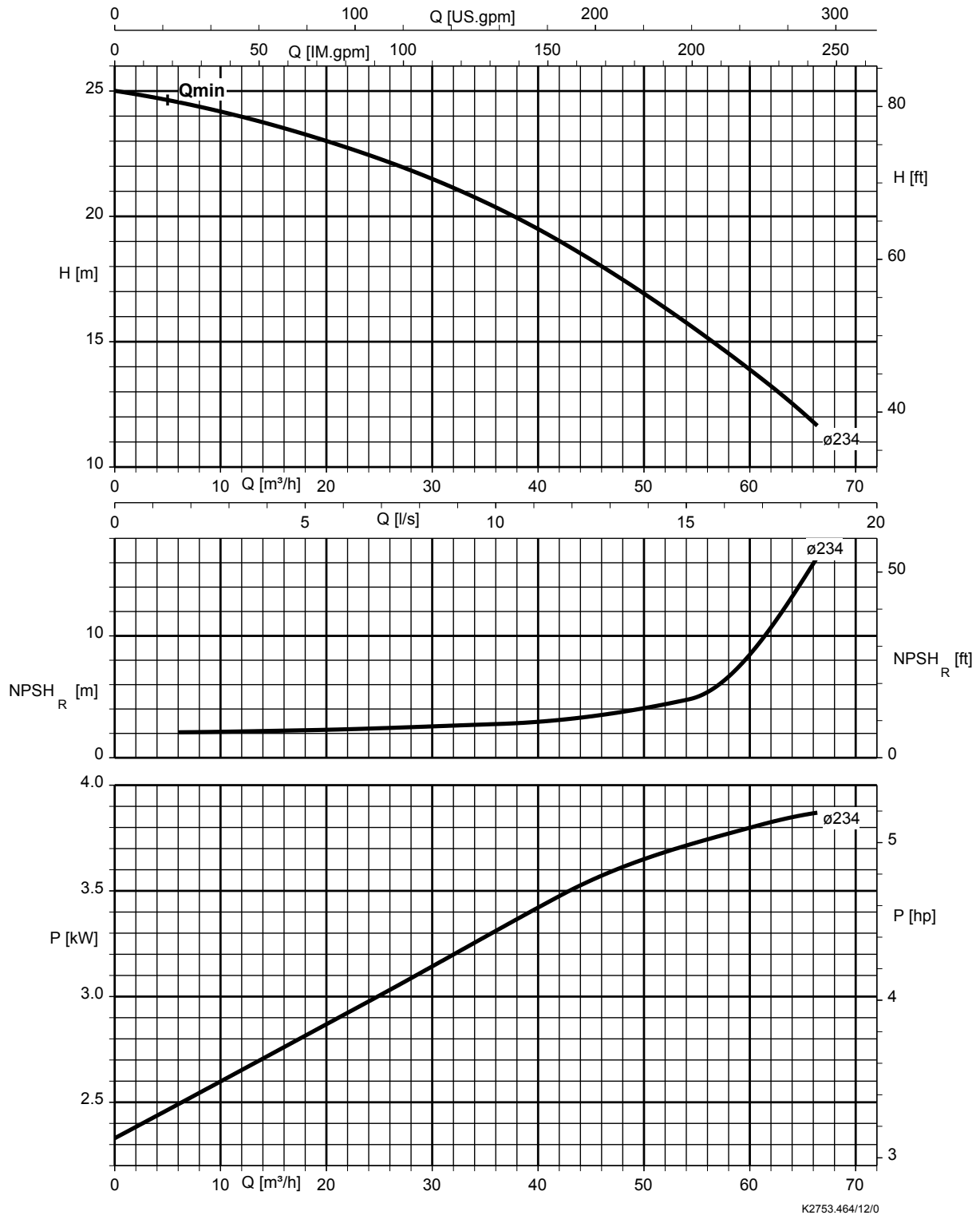
Etaprime L/B 100-100-240.1, n = 1750 rpm
